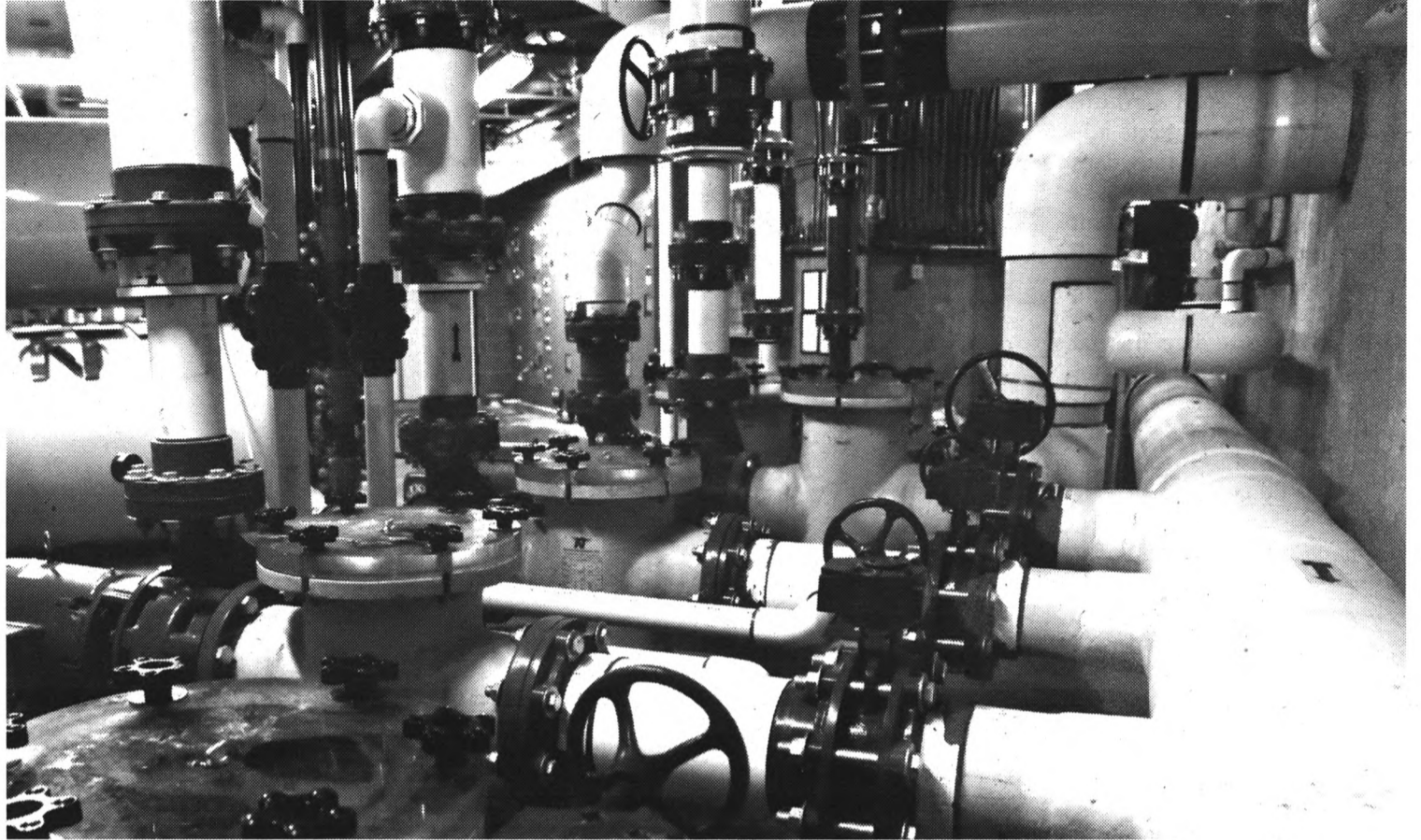
Le système de filtration de la piscine du Centre des Jeux du Canada.
