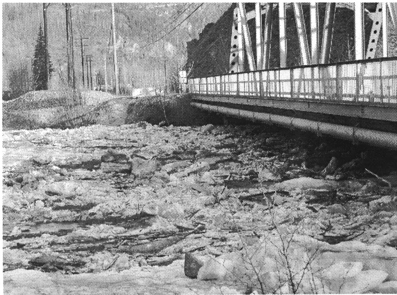
La rivière Klondike a monté jusqu'à environ un mètre de ce tablier de pont durant l'inondation d'avril 2003. Photo : R. Janowicz
