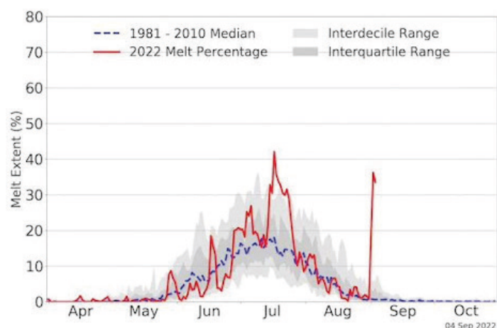
Étendue de la fonte (en % de la superficie). En bleu: médiane 1981-2010. En rouge: 2022.
